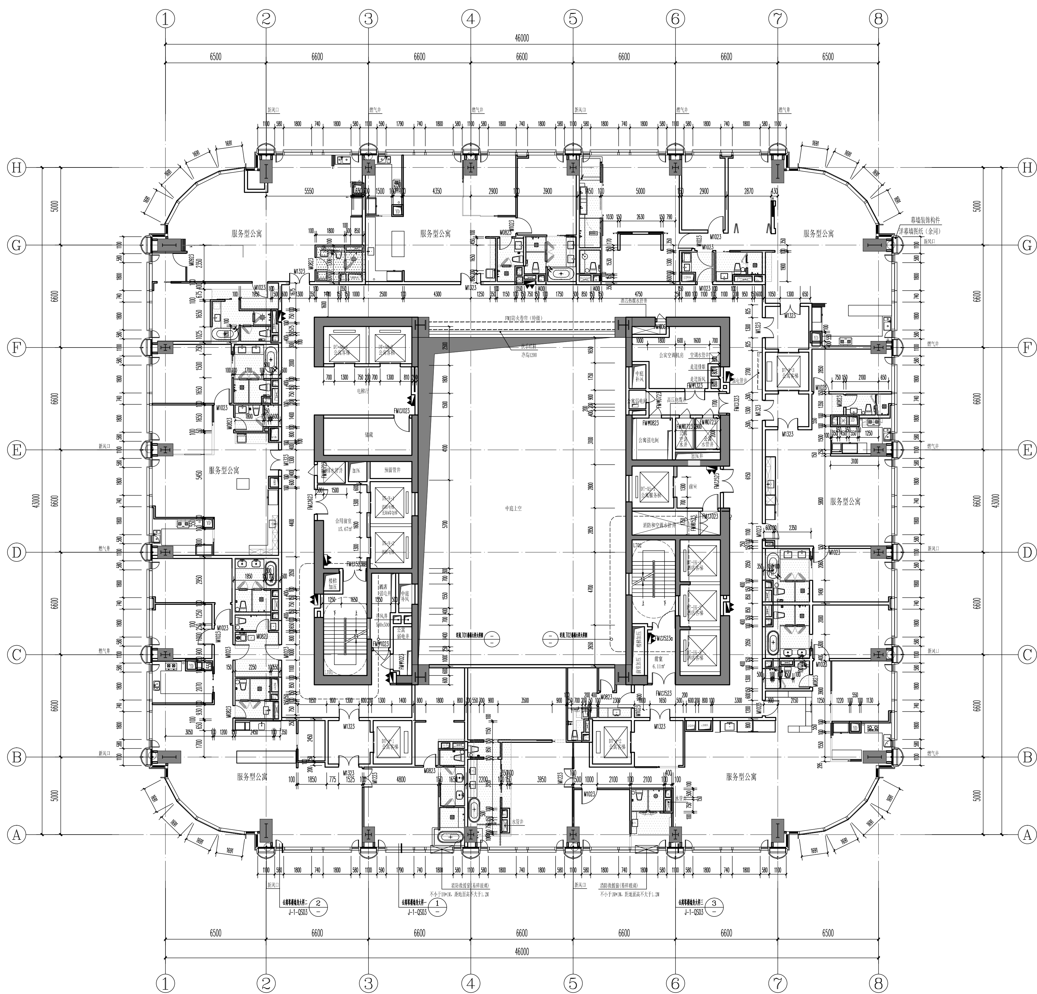
四十一~四十三层层平面图 1:150
